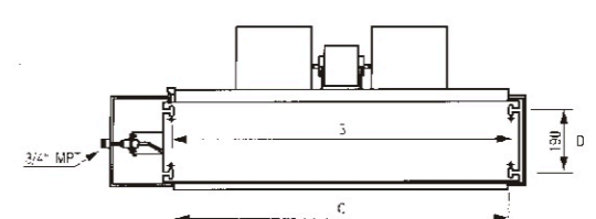
A:機體總長 B:吊孔長度 C:出風口寬度 D:吊孔寬度
